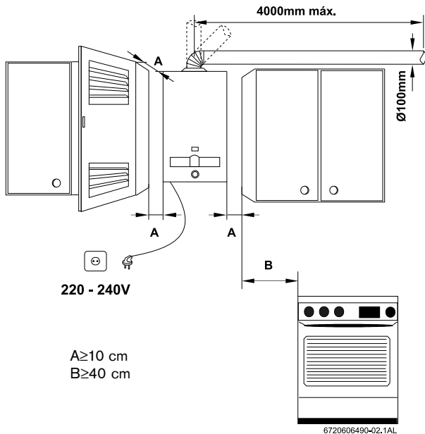
Fig. 4 Distâncias mínimas
